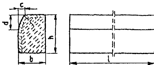
Rys. 1. Wymiarowanie krawężników
